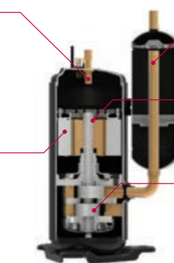
Sprężarka inwerterowa Twin Rotary
