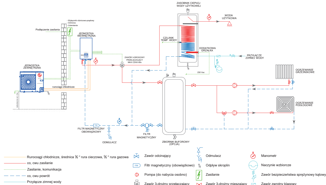
SCHEMAT HYDRAULICZNY
